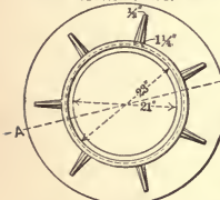
FIG. 7. BROOKLYN, (N. Y.) MANHOLE COVER, 1896.
